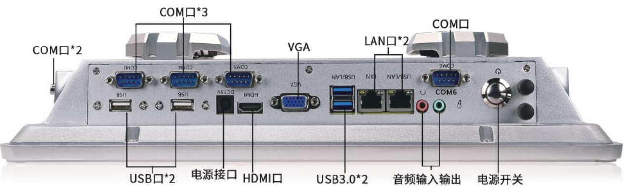
安卓主板接口图
