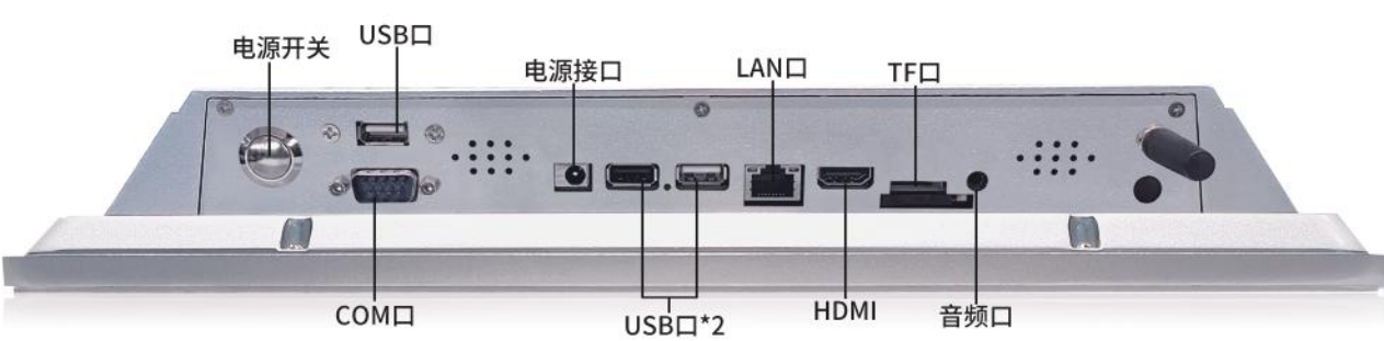
显示器接口图
