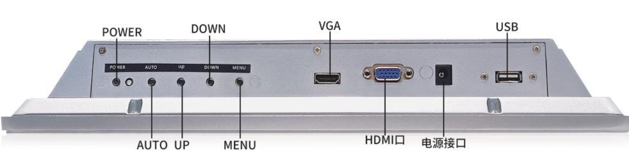
显示器接口图
