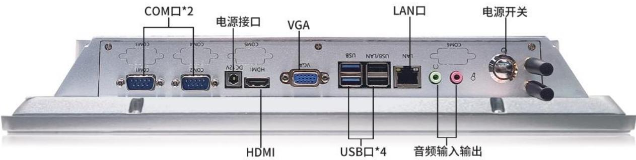
独立酷睿主板接口图
